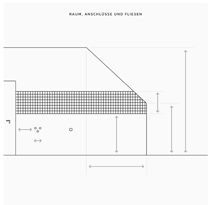
Zu messen: Raumhöhe, eventuelle Dachschrägenhöhe, Abstand von Fliesen zu Boden und Fliesenhöhe. Einzeichnen von Herdanschluss, Wasseranschluss und Abstände zu anderen Objekten.
