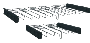
Hostenauszug schmal oder breit mit Vollauszug und Soft-Close-System B/H/T: ca. 37, 83/5/46cm
