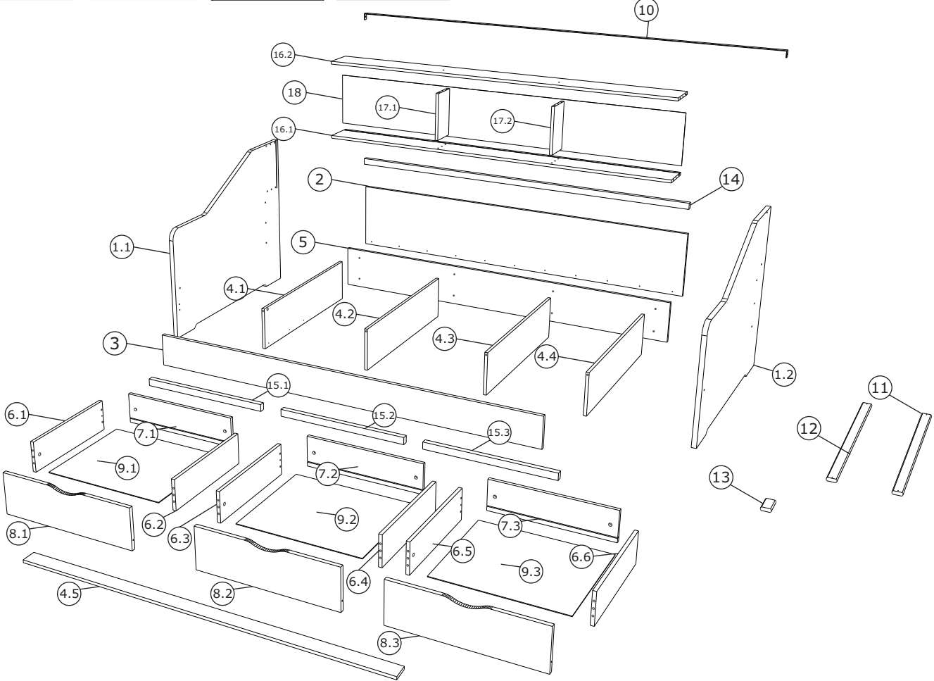
Stückliste / Bill of Materials / Detail visserie
