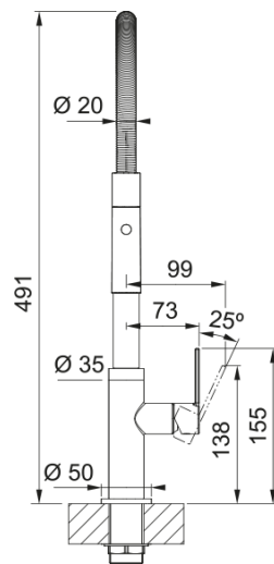
Maris Slim Semi-Pro Zugauslauf Black Matt, Hochdruck, Seitenbedienung, Hebel rechts, Laminarstrahl
