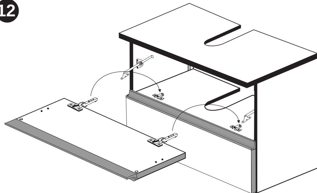
Scharniermontage
