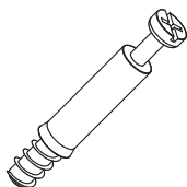
J x24 Ø6x40mm
