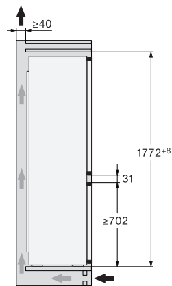
KFN7714F, KFNS7716FC, KD7714E, KD7724E, KDN7714E, KDN7724E Active, Seitenansicht (Skizze)
