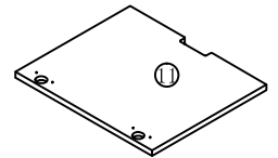
415*348*15mm 1PC
