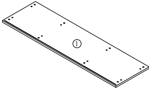
1200*350*15mm 1PC
