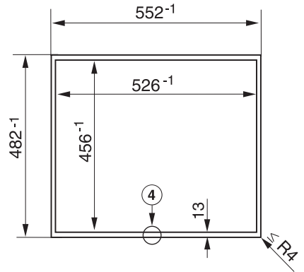
KM 6017 (Skizze)
