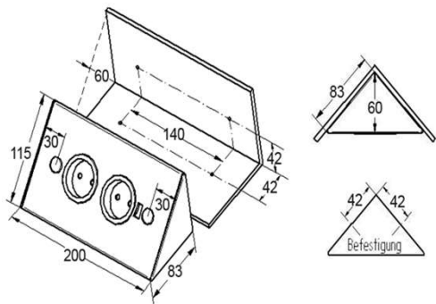
Maßzeichnung dimensioned drawing
