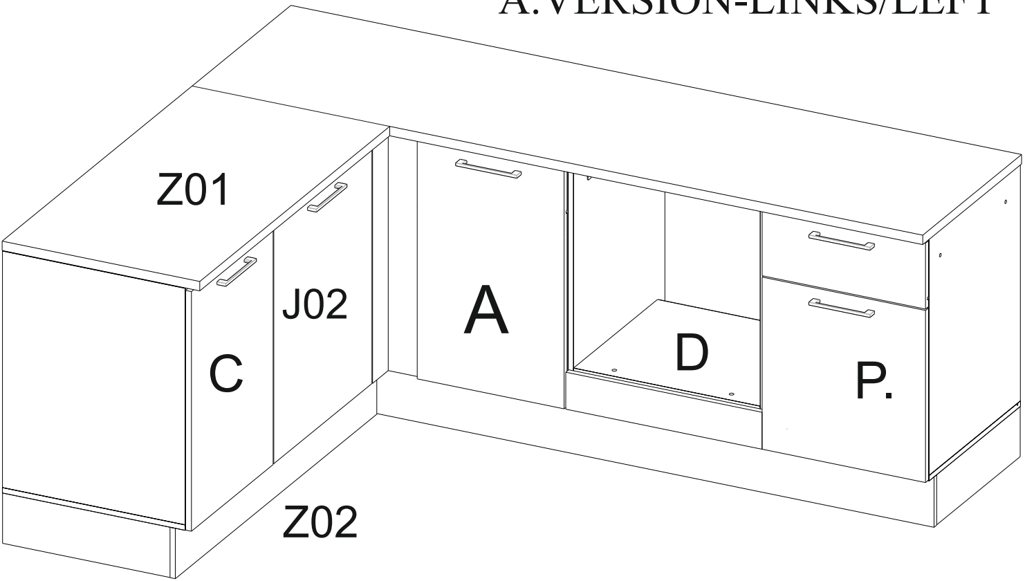
A.VERSION-LINKS/LEFT
