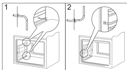
Einsetzen der Blechträger
