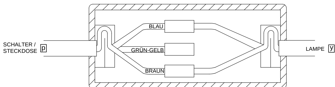
T16 ANSCHLUSSDOSE
